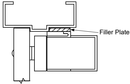
FIG. 2B Filler Plate
